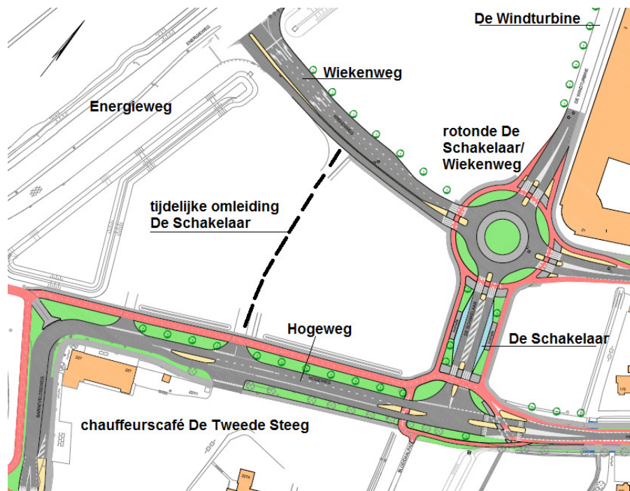
Figuur: situatie met tijdelijke omleiding De Schakelaar en de geprojecteerde rotonde
